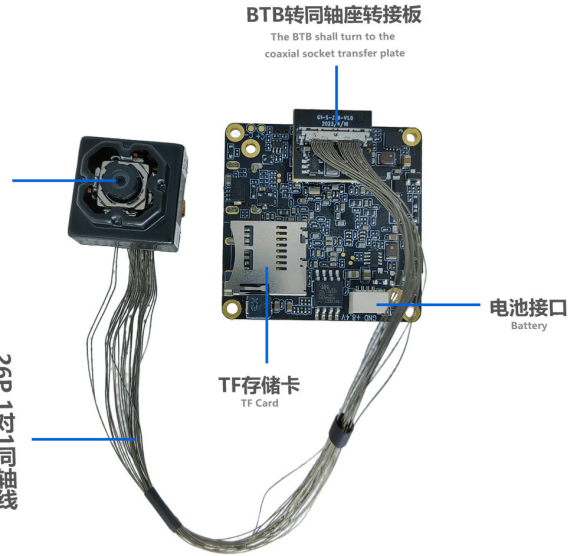
Sony IMX258 光学防抖模组 OIS Anti-shake module
